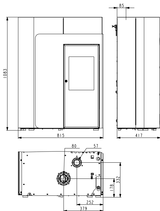
HSP 8 VOLTERRA II perl-schwarz, weiss 05 445 08 25 0000 EAN 90 027 42 48 8062
