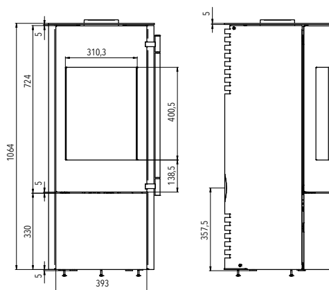
LURE MIT TOPPLATTE Speckstein für LURE und LURE HSC* Gewicht: 27 kg
