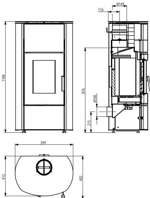
VILORA.HSC* perl-schwarz, mit Holzfach 03 010 10 28 0000 EAN 90 027 42 48 6358
