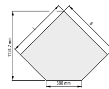
GLASPLATTE MIT ABGESCHRÄGTER KANTE 45° 1000 x 1000 x 580 mm 11 155 10 20 0000 EAN 90 027 42 32 9785
