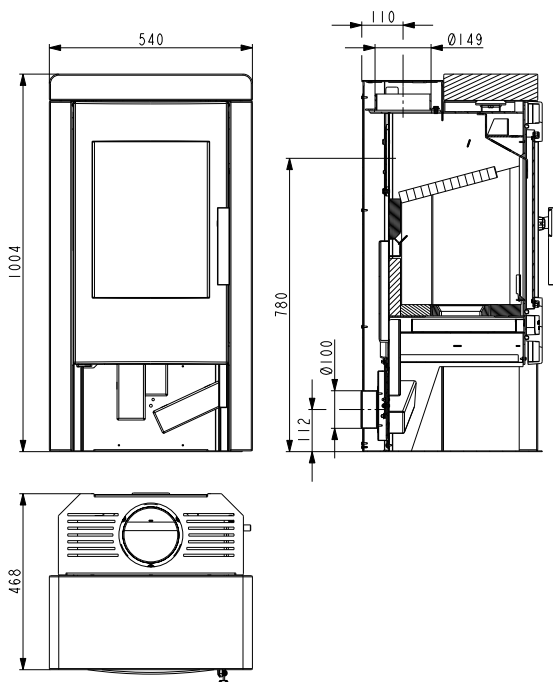
PYRUS EASY HSC perl-schwarz, Stein Speckstein, mit Holzfach 04 294 15 14 0000 EAN 90 027 42 46 1751
