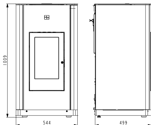
HSP 6 PELLETTO-IV perl-grau, perl-anthrazit 05 419 08 17 0000 EAN 90 027 42 46 0754
