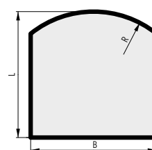
GLASPLATTE SEGMENTBOGEN UND DEKOR-RAHMEN 1000 x 1000 / R = 800 mm 11 159 10 32 0000 EAN 90 027 42 43 0214
