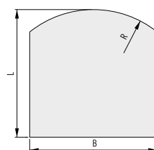
GLASPLATTE MIT SEGMENTBOGEN 1000 x 1000 / R = 800 mm 11 159 10 30 0000 EAN 90 027 42 39 2369
