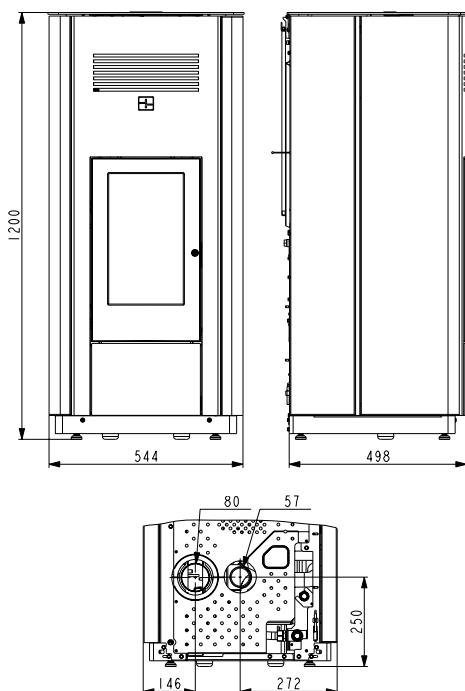
HSP 6 WT RLU perl-anthrazit, perl-schwarz 05 537 08 04 0000 EAN 90 027 42 46 2765
